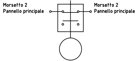
Galleggiante elettrico
